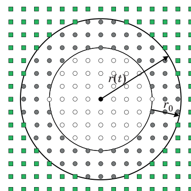
■ Рис. 2. Модель распространения критичного сообщения в сети VANET
