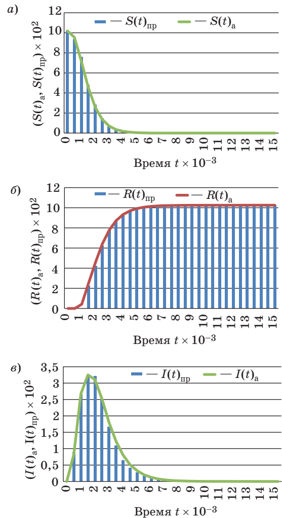
■ Рис. 5. Диаграмма изменения средней численности восприимчивых (а), восстановившихся (б) и инфицированных (в) узлов
