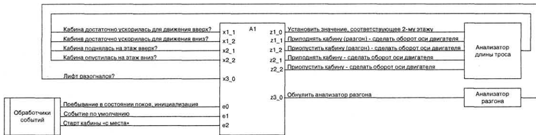
■ Рис. 3. Схема связей автомата A1. Управление двигателем, перемещающим лифт между этажами
