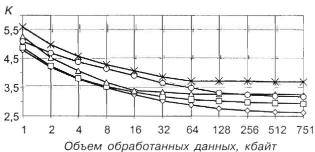
■ Рис. 1. Изменение K по мере обработки book1 при V = 64 кбайт: —◇— PPM 3-1-0(A); —□— PPM 2-1-0(A); —△— bzip2*; —○— LZari; —*— LZW
